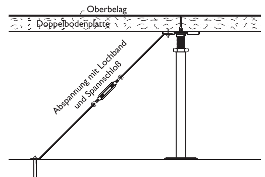
Abspannung Plattenreihe
