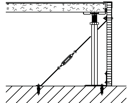
Abspannung Frontverkleidung
