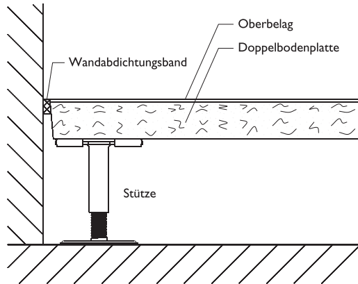
Wandanschluß
